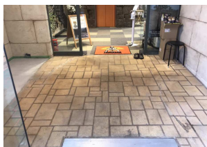
⑤ 3層目：表層吹き付け
